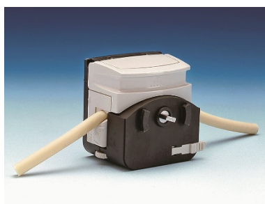
313X(X2)型ヘッド
